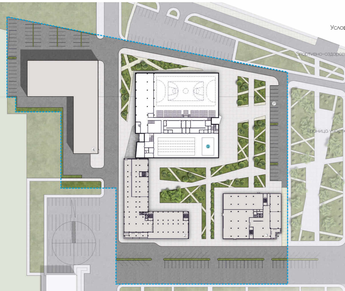
Схема генплана
