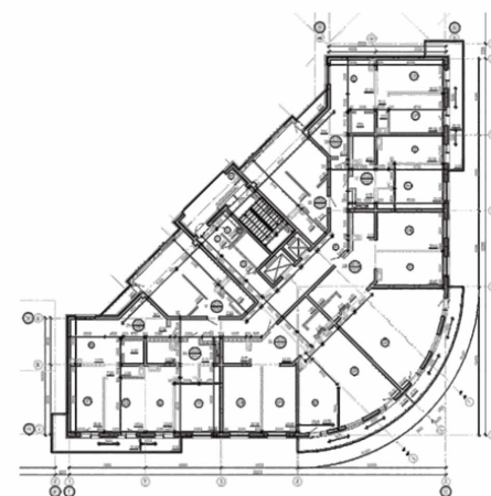
План типового этажа 2-18 эт.
