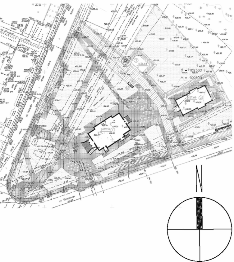
Схема генплана
