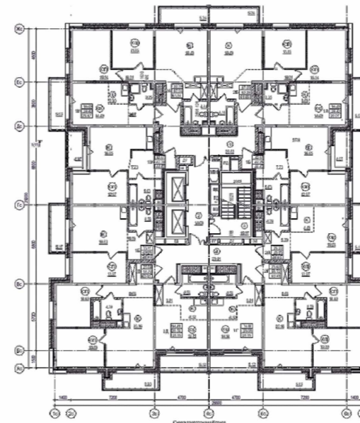
План типового этажа
