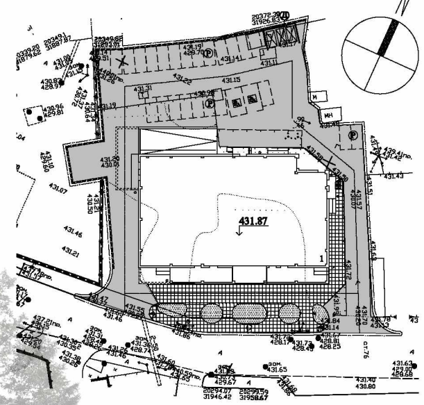
Схема генплана
