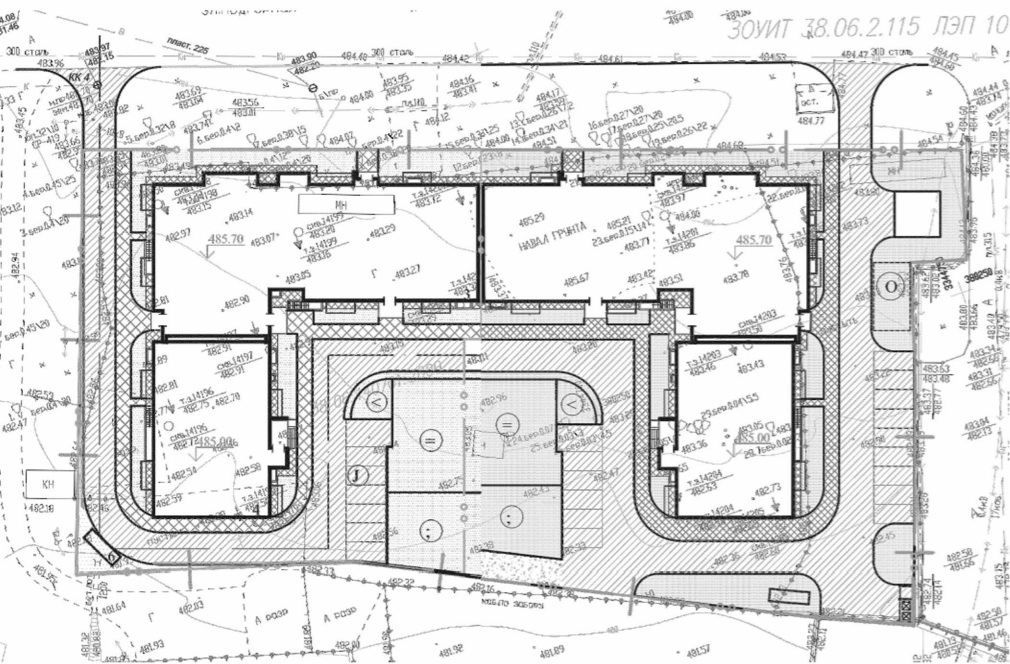
Схема генплана
