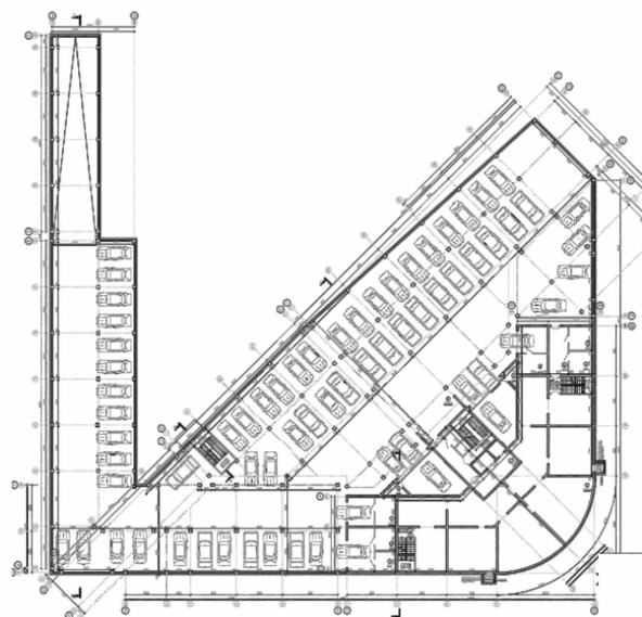
План подвала на отм. -7.800
